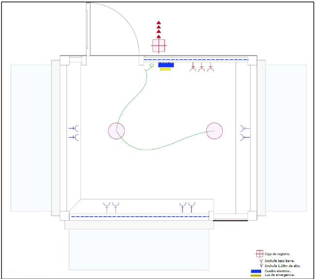
Esquema electricidad almacén .
